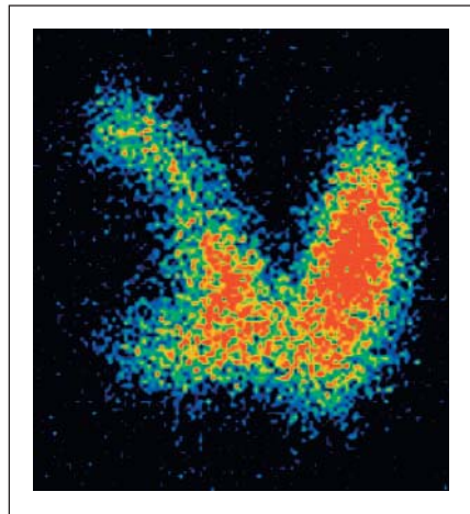
Abb. 2.7: Szintigraphie mit ^{99m}\text{Tc} : „Kalter“ Knoten: Der sonographisch solide Knoten rechts zeigt szintigraphisch eine fehlende Aktivitätsaufnahme im Sinne fehlender Hormonproduktion.
